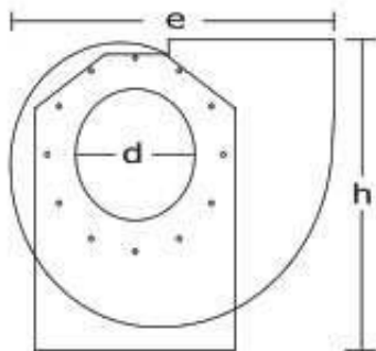
Φ350-5.5HP-1450RPM
